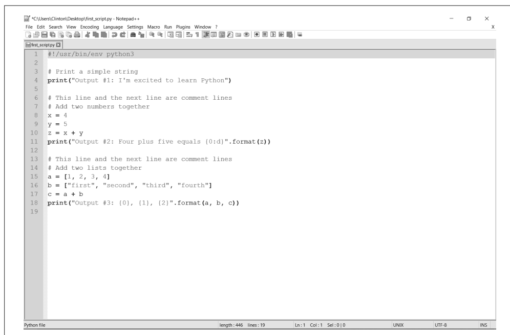
图 1-8: 在 Notepad++ (Windows) 中为 first_script.py 添加新代码
