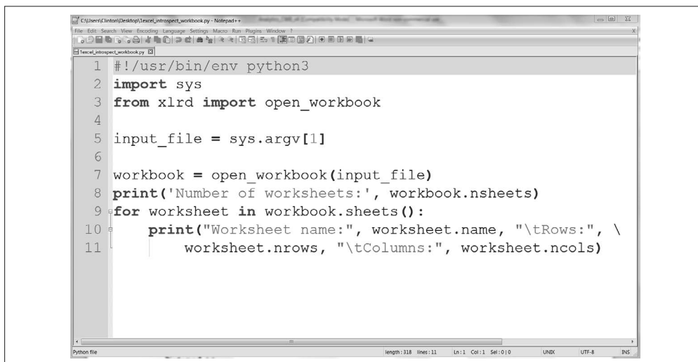
图 3-5: Notepad++（Windows）中的 Python 脚本 1excel_introspect_workbook.py
